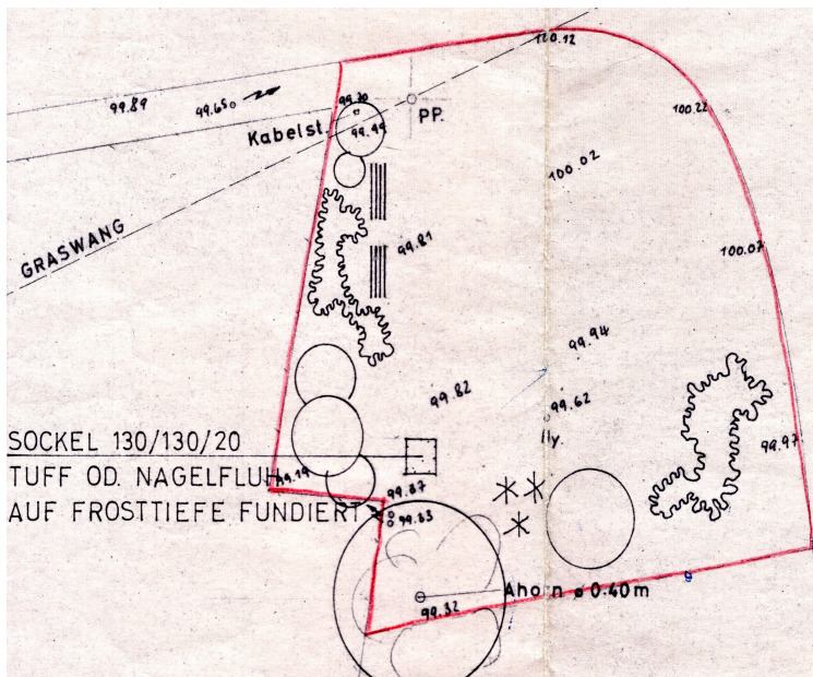
Bauplan "Rastplatz Graswang"
